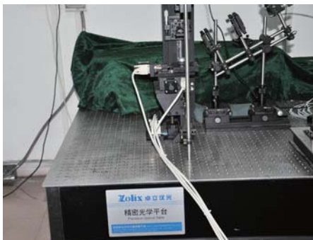
华南理工大学隔振平台及电动滑台
